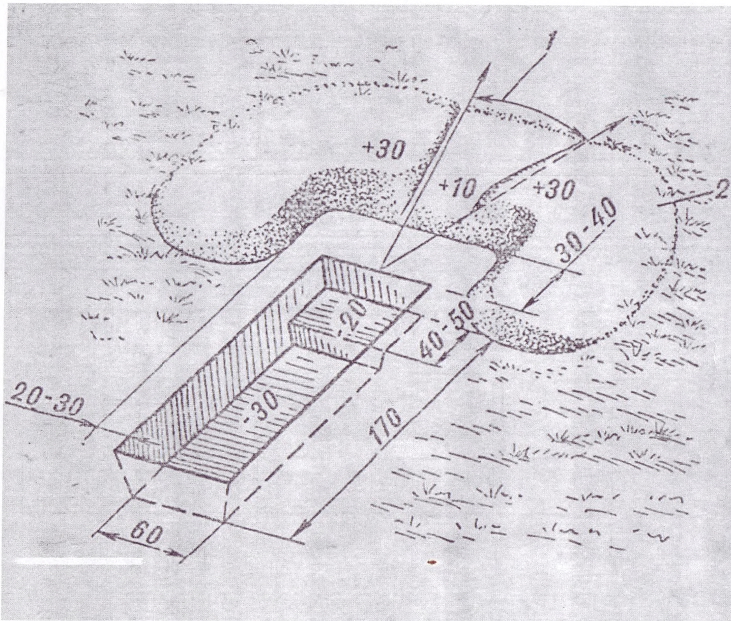
Рис. 21 Одиночный окоп для стрельбы из автомата лежа: 1 сектор обстрела; 2 бруствер
